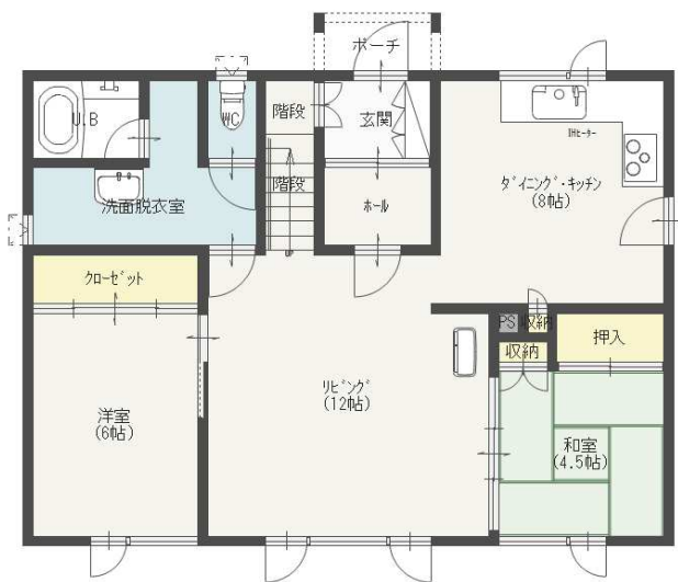
1F平面図
