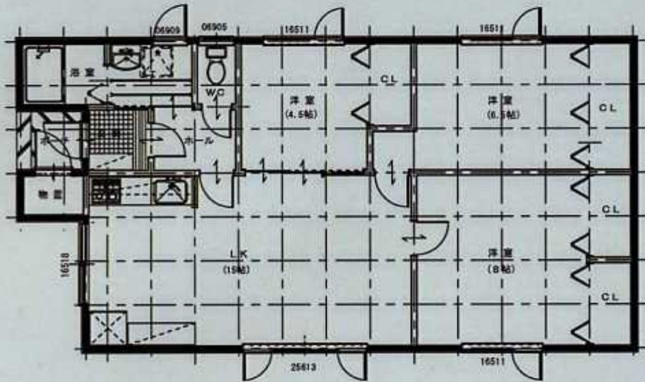
平面図
